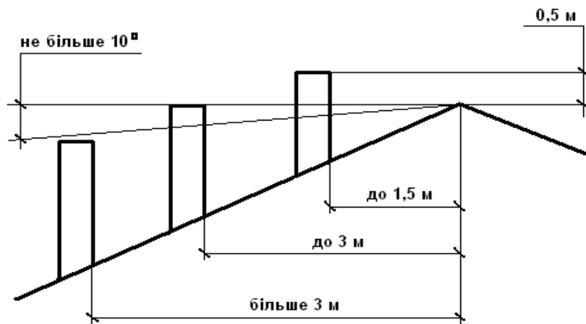
Рисунок 4. Розміщення димоходу
