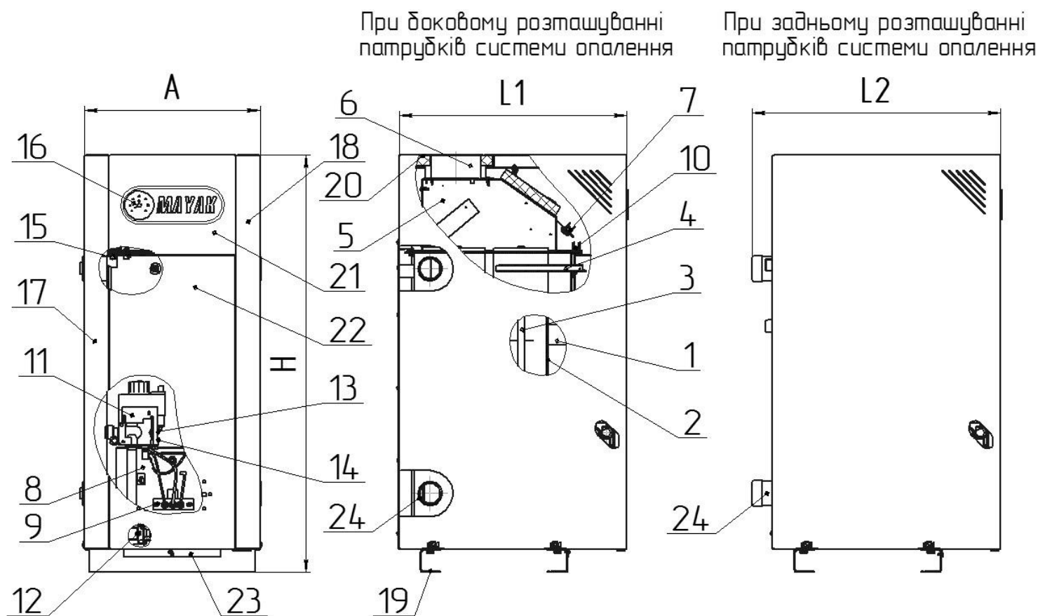
Рисунок 1. Котел опалювальний сталевий
