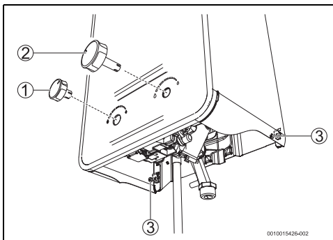
Мал. 17 Зняття передньої частини кожуха
