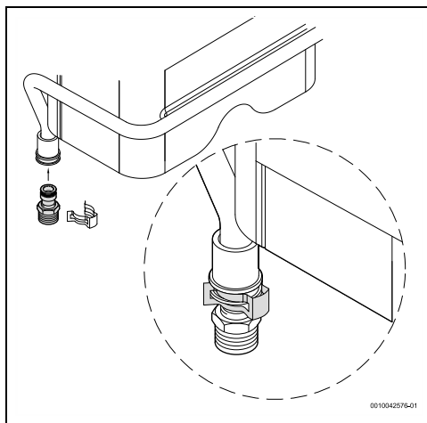
Мал. 13 Адаптер
