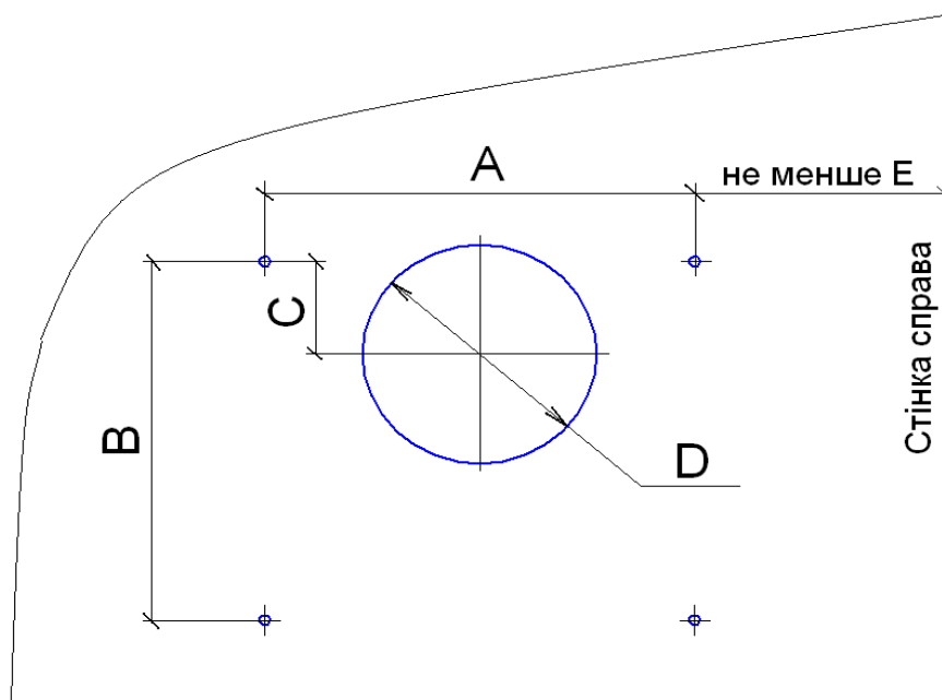
Рисунок 4. Монтажні розміри котлів
