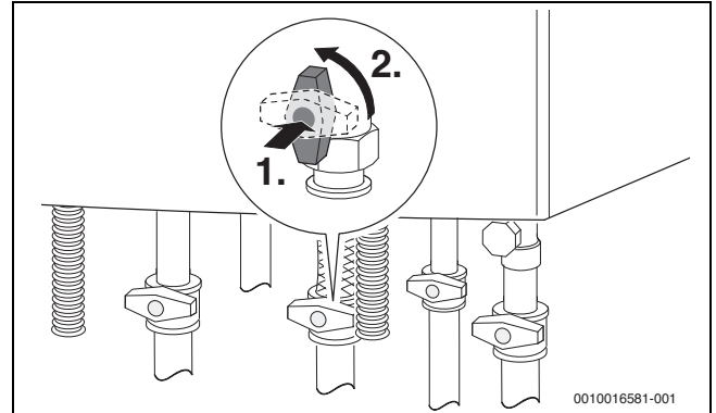
Мал. 3 Відкриття газового крана
