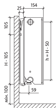
тип RCVM 33
