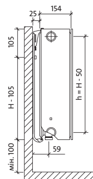
тип FCVM 33
