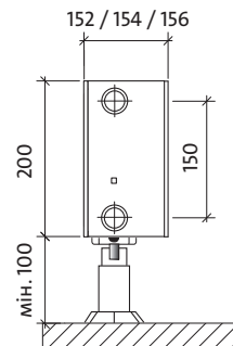
тип 33
