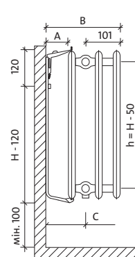
тип HV 30
